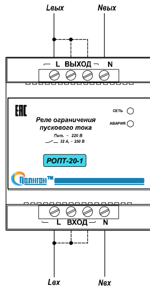
Рис.1 Схема подключения модуля к сети с рабочим током до 20 А.
