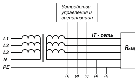
Рис.2. Типовая схема подключения блока РКИ-500-50 к трехфазной сети с нейтралью.
