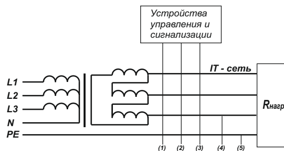
Рис.3. Типовая схема подключения блока РКИ-500-50 к трехфазной сети без нейтрали.
