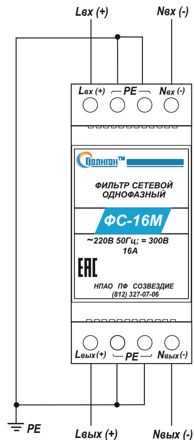
Рис.1. Порядок подключения фильтра ФС-16М.
